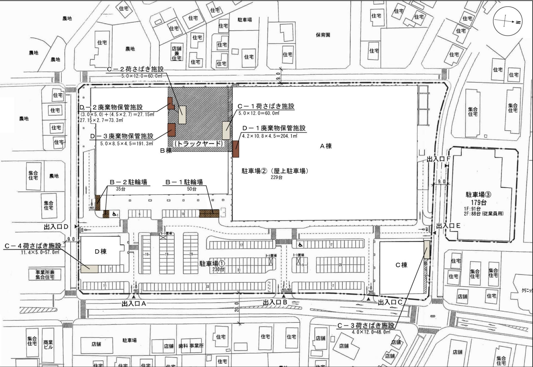
建物配置図（変更前）
